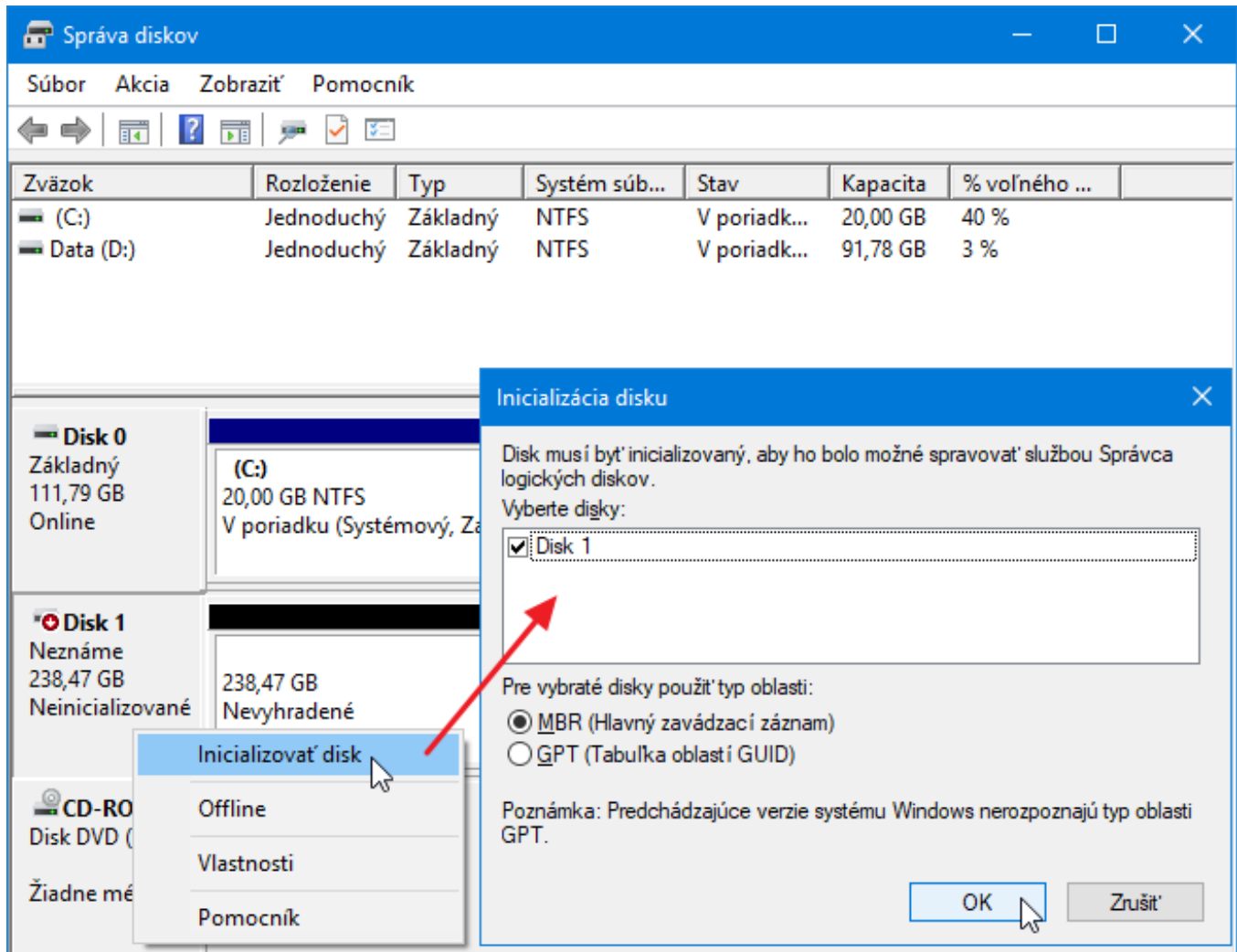
OBRÁZOK 2. Inicializácia disku.
